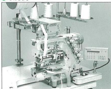
◎ 偏平縫いミシン (VG2700クラス) への AEF-31 取付例
