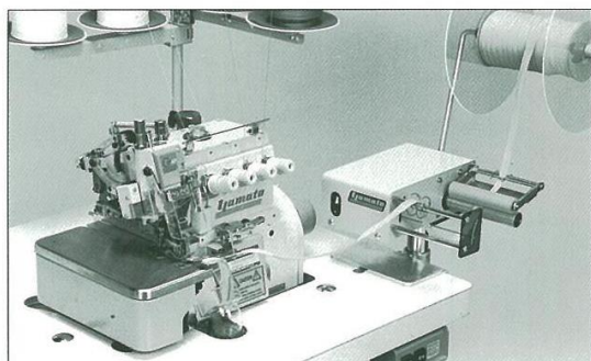
◎ 偏平縫いミシン (VG2700クラス) への AEF-31 取付例
